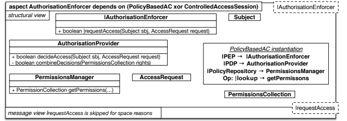
Fig. 10. Aspect AuthorisationEnforcer
